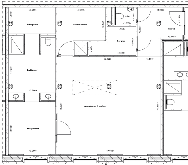
Plattegrond verdieping 01 1:50
